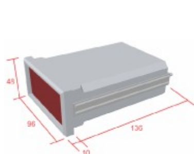
UNIDADE ELETRÔNICA CAIXA 48 x 96 mm RECORTE DO PAINEL: 43 x 91 (+/- 1 mm)
